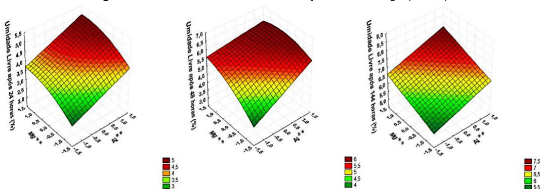
Figura 5. Umidade do GTSP com a variação de Al^* e Mg^* ( Fe^*=0 )
