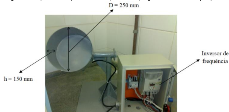
Figura 1. Aparato experimental (bancada) - granulador do tipo prato
