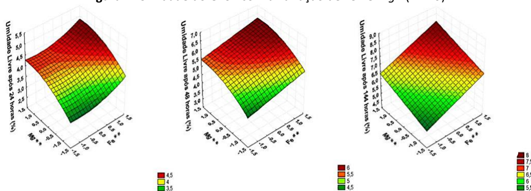
Figura 4. Umidade do GTSP com a variação de Fe^* e Mg^* ( Al^*=0 )
